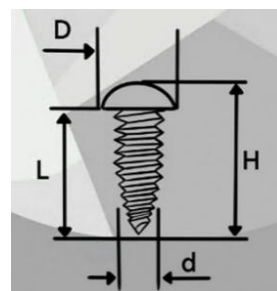
Rys. 1 wymiary śruby
